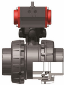
Шаровой кран общего применения ХПВХ с пневмоприводом НО с муфтовыми окончаниями d90 (DN80)
