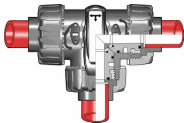
3-х ходовой шаровой кран ТКД с муфтовыми окончаниями L-шар (уплотнение FKM) PP-H d63 (DN50)
