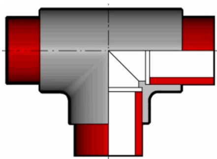
Тройник ПВДФ 90° d16 SDR21 PN16
