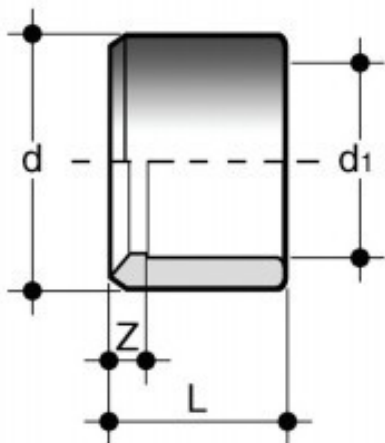
Переходное кольцо ХПВХ 32х25 PN16
