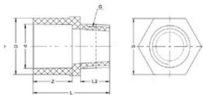
Муфта переходная для раструбной сварки с НР РР-Н IPS d50 PN10
