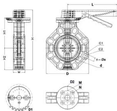
Затвор дисковый ХПВХ с рукояткой FKM IPS d110 (DN90)
