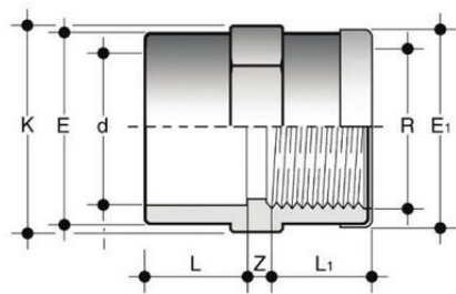
Переходная муфта с усиливающим кольцом ХПВХ 63x2" PN16
