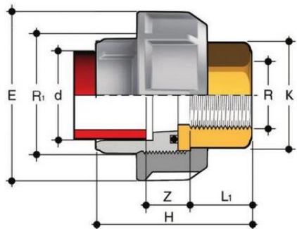
Муфта разборная переходная РР-Н / латунь, ВР (EPDM) FIP 32x1 PN10
