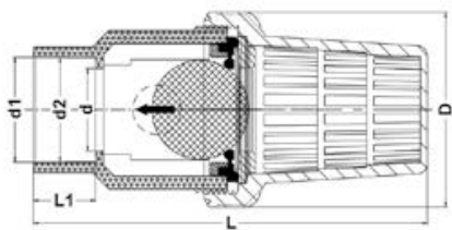
Донный клапан IVZ ПВХ с муфтовыми окончаниями, FKM, FIP d90 (DN80)
