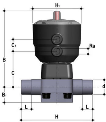
Мембранный клапан ДК ПВДФ с пневмоприводом НЗ, PN10 с втулочными окончаниями d32 (DN25)
