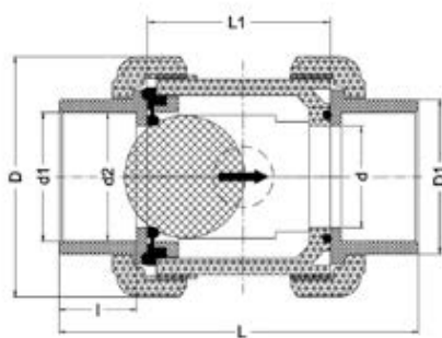
Шаровой обратный клапан ISXE ПВХ; с муфтовыми окончаниям, EPDM, IPS d90
