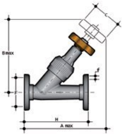
Угловой вентиль VVOV ПВХ с фланцевыми окончаниями, EPDM, FIP d25 (DN20)
