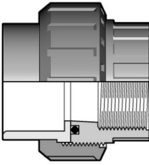
Муфта разборная с ВР ПВХ FIP 32x1
