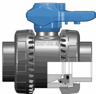
Шаровой кран ПВХ общего применения VEE; муфтовые окончания, EPDM, FIP d20 (DN15)
