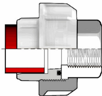
Муфта переходная разборная НР ПВДФ 63х2 SDR21 PN16
