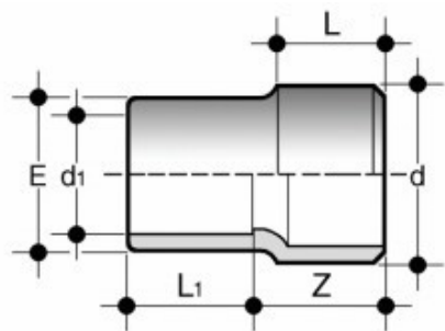
Втулка редукционная ПВХ FIP 20x16
