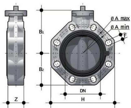
Дисковый затвор ПВХ FKOAVFM со свободным штоком, FKM, FIP 16"
