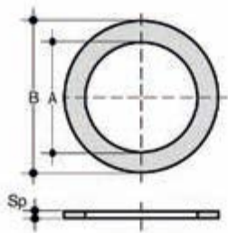
Плоское уплотнение IPS под фланцевое соединение (FKM) d140
