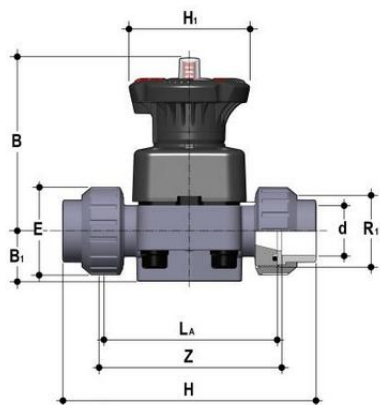
Мембранный клапан ДК ХПВХ с разборными муфтовыми окончаниями d32 (DN25)
