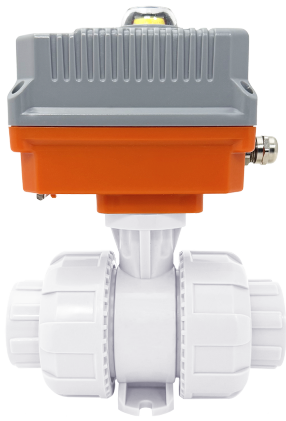
Шаровой кран IVKD ПВДФ с эл.приводом 220V AC, муфтовые окончания, FKM, IPS d50 (DN40)
