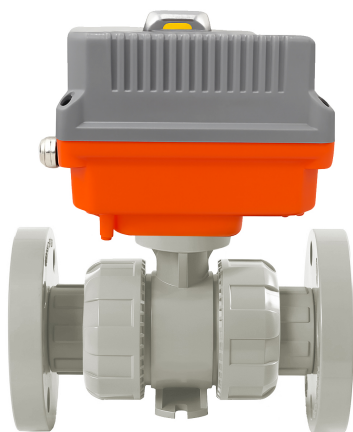
Шаровой кран IVKD ПП-гомополимер с эл.приводом 24V DC, фланцевые окончания, EPDM, IPS d25 (DN20)
