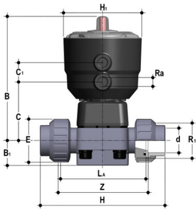
Мембранный клапан ДК ПВДФ с пневмоприводом НО, PN10 с муфтовыми окончаниями d40 (DN32)
