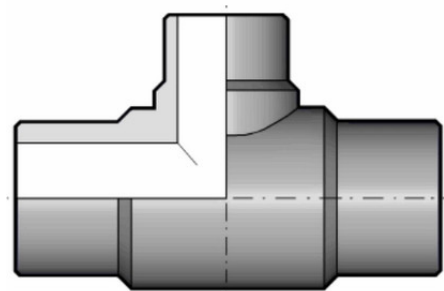
Тройник редукционный для стыковой сварки PP-H FIP (PN6) 180x125 SDR17.6 PN6
