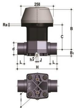
Мембранный клапан VM с пневмоприводом H3 с втулочными окончаниями (уплотнение FKM/мембрана FKM) PP-H d90 (DN80)
