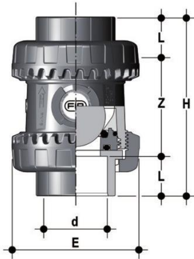
Шаровой обратный клапан SXEIV ПВХ; с муфтовыми окончаниям, ФКМ, FIP d110 (DN100)
