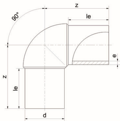
Отвод 90° PP-H Simona d110 SDR11 PN10
