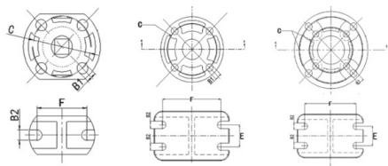
Шаровой кран IVKD ПП-гомополимер с эл.приводом 220V AC, муфтовые окончания, EPDM, IPS d40 (DN32)
