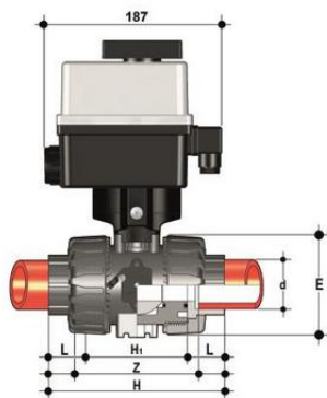
Шаровой кран для регулирования потока VKR ПВДФ с эл.приводом 90-240V, муфтовые окончания d63 (DN50)
