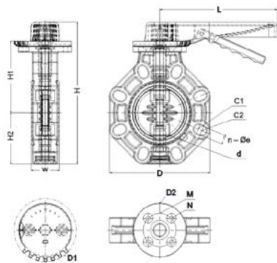
Затвор дисковый ПВХ с рукояткой промышленного применения EPDM IPS 140 (DN125)
