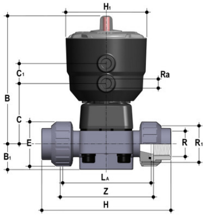
Мембранный клапан ПВХ с пневмоприводом, PN10, DK, EPDM, FIP R2" (DN50)
