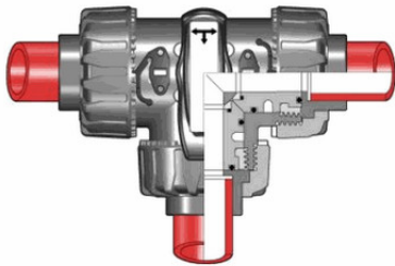
3-х ходовой шаровой кран ТКД с муфтовыми окончаниями L-шар (уплотнение EPDM) PP-H d63 (DN50)
