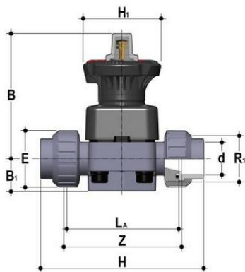
Мембранный клапан DK/L ПВХ с муфтовыми окончаниями d20 (DN15)
