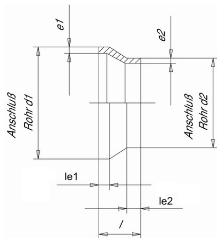
Муфта редукционная ПВДФ (Simona) 90x63 SDR33 PN10
