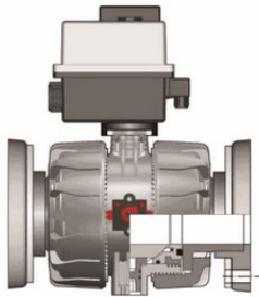
Шаровой кран VKD с эл.приводом 90-240V, фланцевые окончания, DN65-100 (уплотнение FKM) PP-H d75 (DN65)
