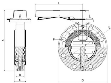
Затвор дисковый ХПВХ с рукояткой EPDM Comer d160 (DN150)
