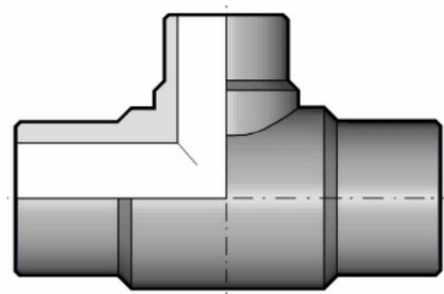
Тройник редукционный для стыковой сварки PP-H FIP 180x110 SDR17.6 PN10
