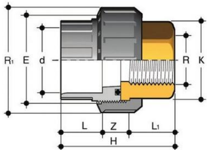
Муфта разборная ХПВХ/ латунь, ВР 25x3/4" PN16
