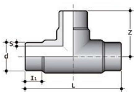
Тройник равнопроходной для стыковой сварки PP-H FIP d90 SDR11 PN6
