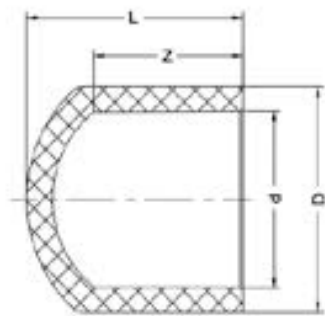
Заглушка ПВХ для раструбной сварки d63 PN 16
