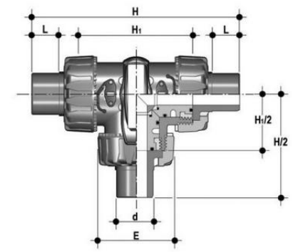
3-х ходовой шаровой кран ТКД с втулочными окончаниями L-шар (уплотнение FKM) PP-H d50 (DN40)
