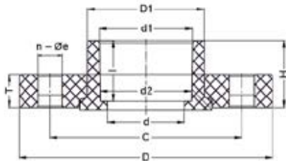
Фланец свободный с буртом ХПВХ IPS (Model A) d40 PN16
