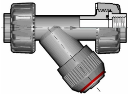
Грязевый фильтр RVUFV PBX с резьбовыми окончаниями, EPDM, FIP 3/4"
