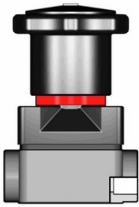
Компактный мембранный клапан CM с муфтовыми окончаниями (уплотнение FKM / мембрана PTFE) PP-H d16 (DN12)
