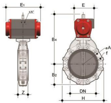
Дисковый затвор промышленного применения FK ПВХ с пневмоприводом, EPDM, FIP d315 (DN300)
