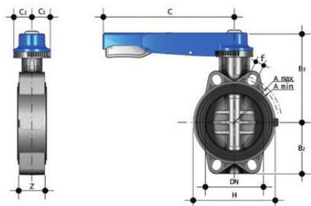
Дисковый затвор ПВХ FEOVLM с рукояткой, EPDM, FIP d140 (DN125)
