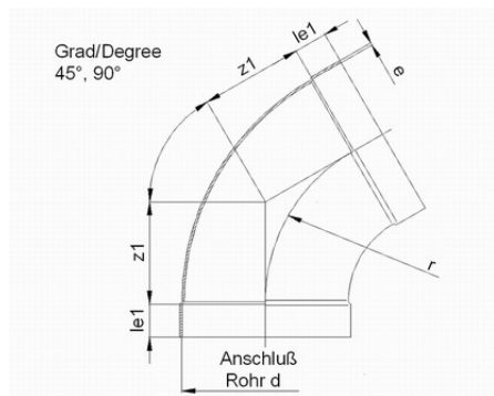
Изгиб 45° PPs d110
