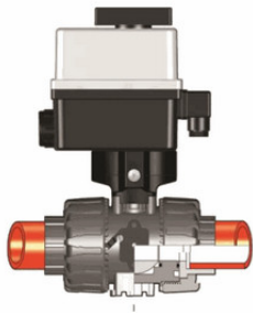
Шаровой кран VKD с эл.приводом 24V AC/DC, муфтовые окончания (уплотнение EPDM) PP-H d32 (DN25)
