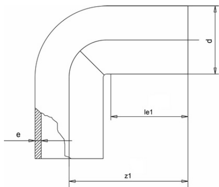
Изгиб ПВДФ 90° (Simona) d63 SDR21 PN16
