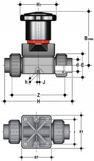
Компактный мембранный клапан CMFV ПВХ с резьбовыми окончаниями, FKM, FIP d15 (DN15)
