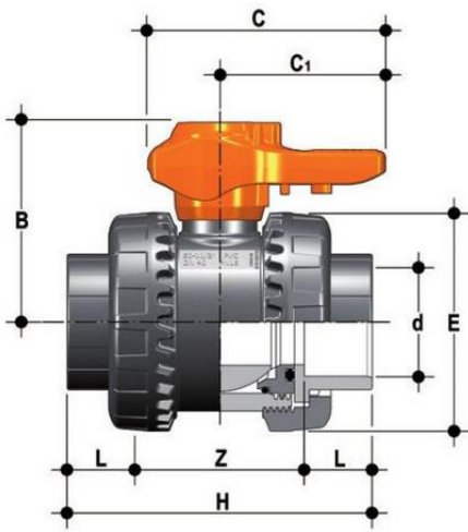
Шаровой кран общего применения VXE ХПВХ с муфтовыми окончаниями d32 (DN25)
